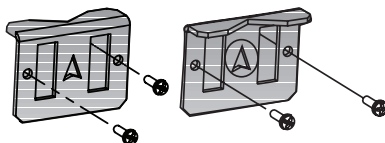
Figura 8: Reorientación de la ménsula superior
