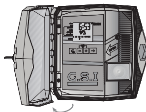
Figura 2: Panel de control girado hacia afuera
