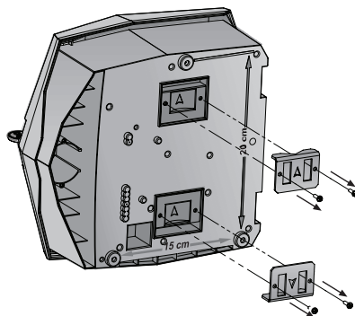
Figura 7: Extracción de las ménsulas de montaje en el poste
