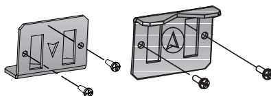
Figura 9: Reorientación de la ménsula inferior
