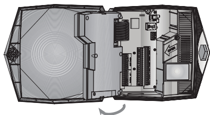
Figura 1: Tapa del controlador abierta
