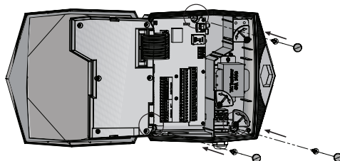
Figura 6: Inserción de los tornillos de montaje con las tapas de cobertura
